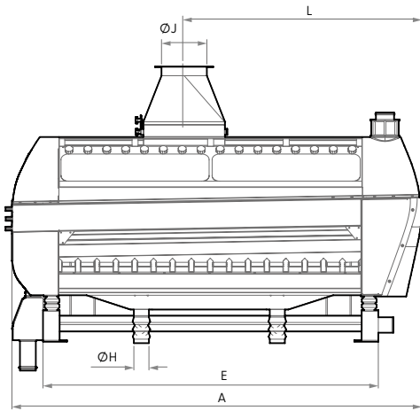
VORDERANSICHT
